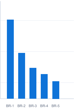
Acidentes e mortos por BR
