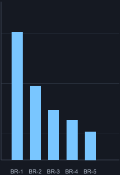
Acidentes e mortos por BR
